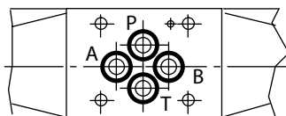
Установочная поверхность ISO 4401 размер O3
