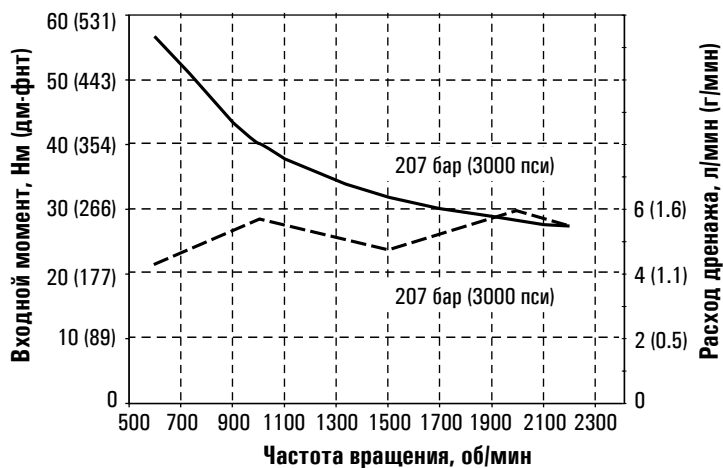
Входной момент и расход дренажа при разгрузке при 49°С (120°С)
