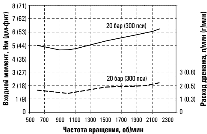
Входной момент и расход дренажа установившийся при 49°С (120°С)
